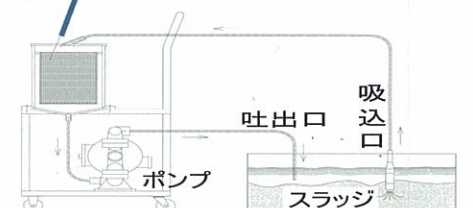
〈装置フロー図〉
